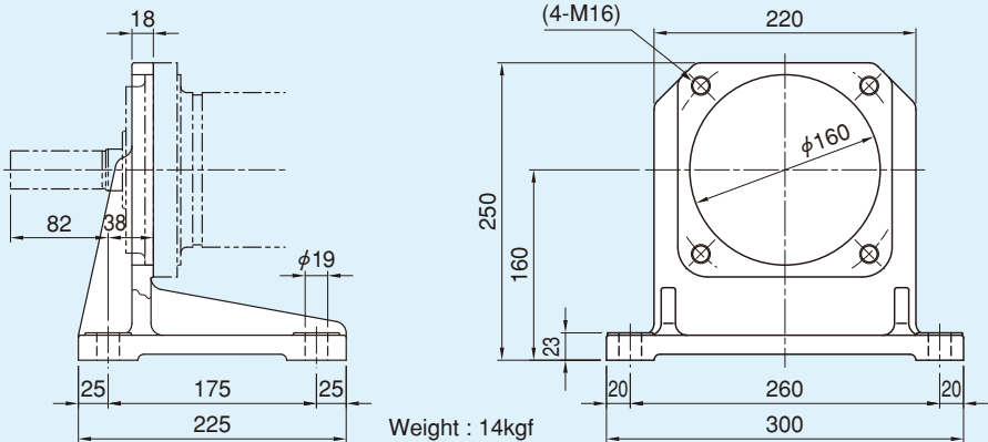
B38,B45-4L用ブラケット Bracket for model B38, B45 品名番号 60BL-B384F
