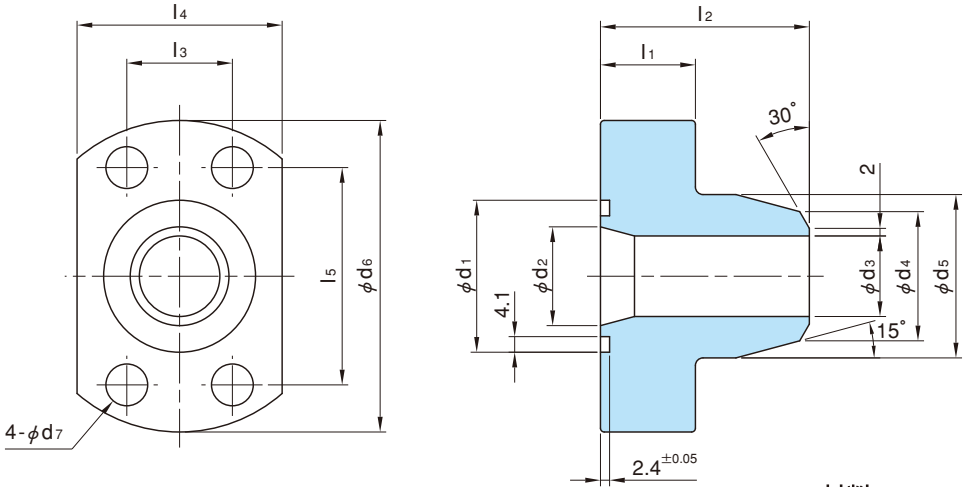
SAE フランジ SAE Flange
